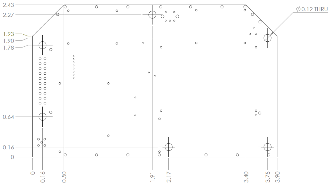
RV-M6, Z50, M50 Miniature Daisy Radio Module
